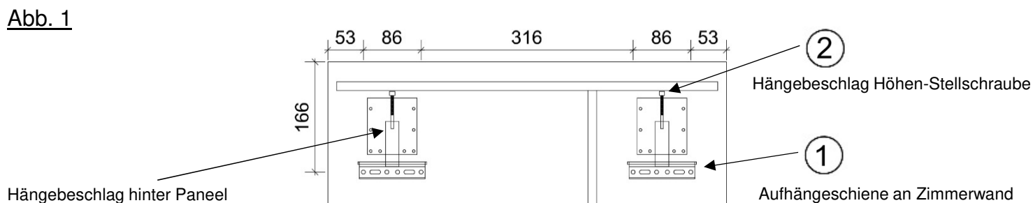
Bohrmaße von Paneel-Außenkanten für Aufhängeschienen
