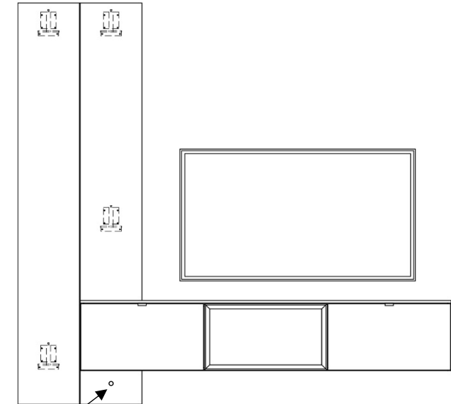
Paneel - Ausschnitt Hängelowboard Höhe: 1 Raster
