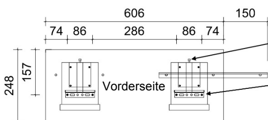
Bohrmaße von Wandboard-Außenkanten für Aufhängeschienen
