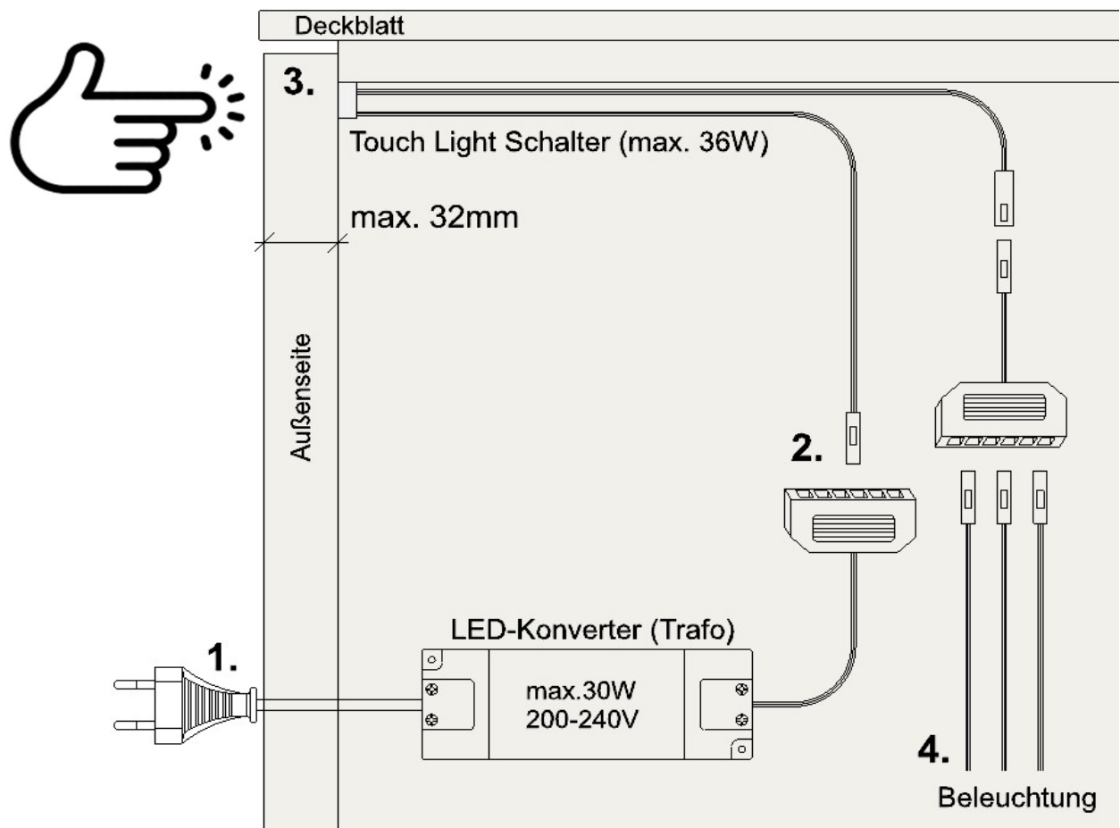
Abbildung 1: Beispiel für Montage hinter dem Möbel
